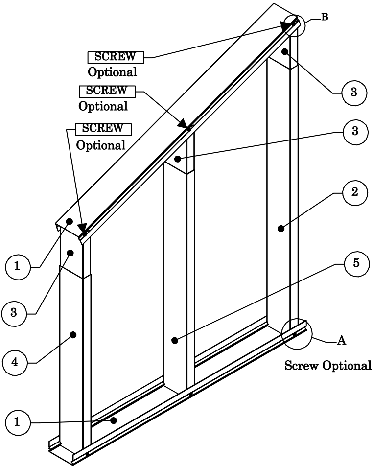
8 STUD RAKE ASSEMBLY
