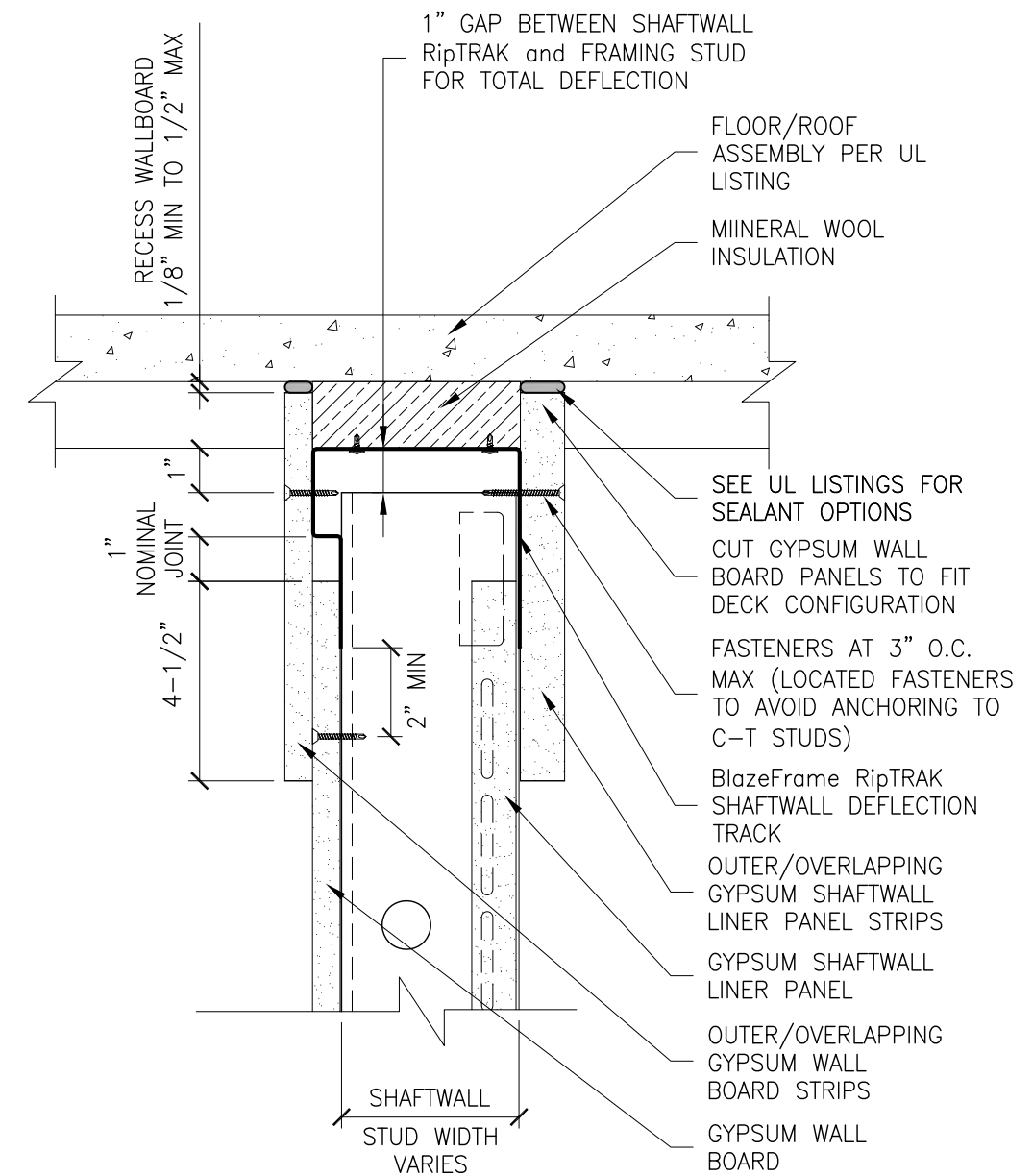
SECTION A-A
